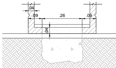
DET 1: Sujeción pata
