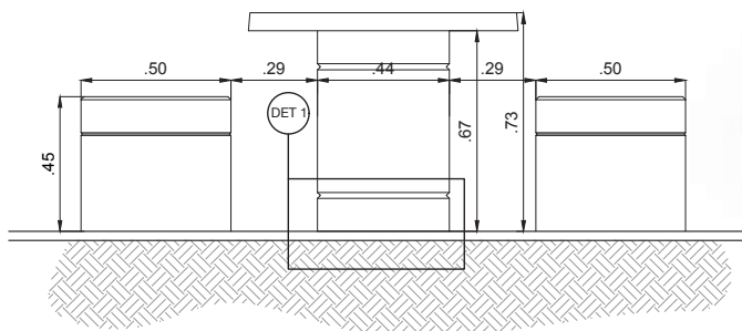
Vista Lateral
