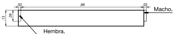
Vista Lateral
