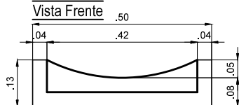
Vista Frente
