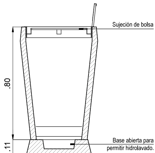
Corte Lateral
